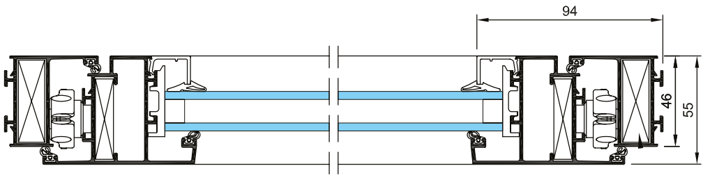
Sección horizontal
