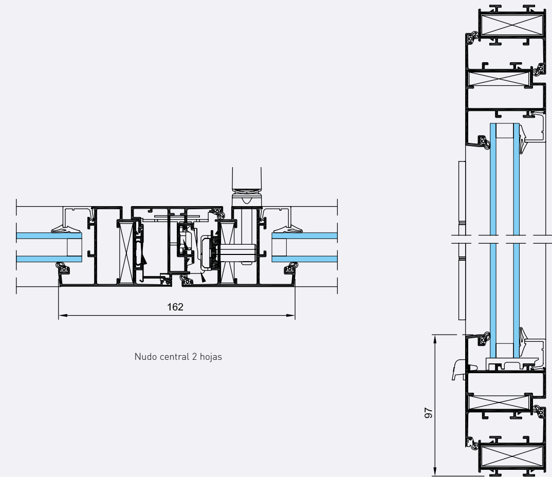
Sección vertical
