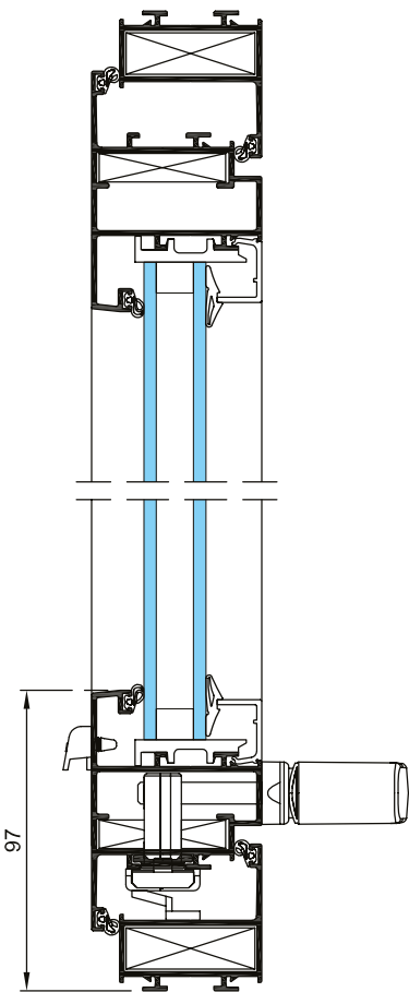
Sección vertical
