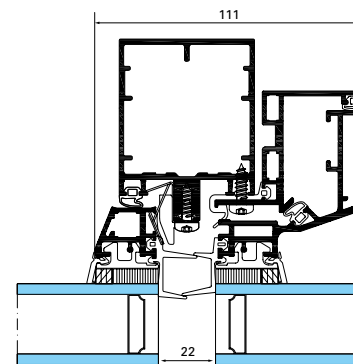
GEODE VEE ventana oculta italiana
