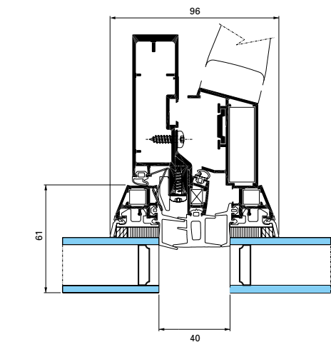
GEODE VEE ventana oculta oscilobatiente
