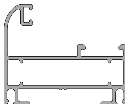
7705 0,821 kg/m
