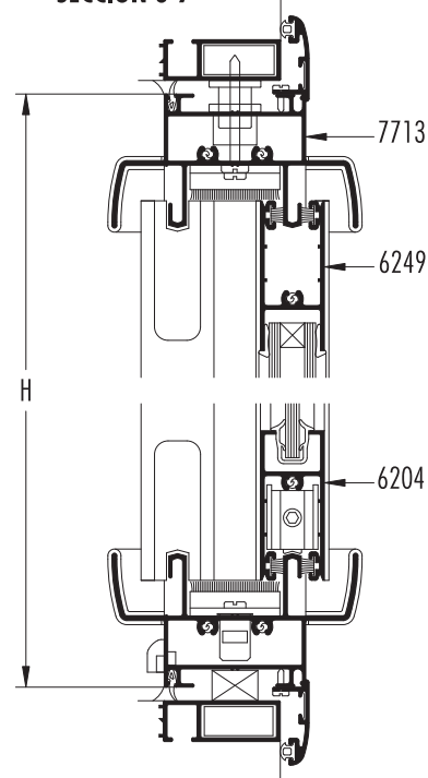
SECCION 6-7
