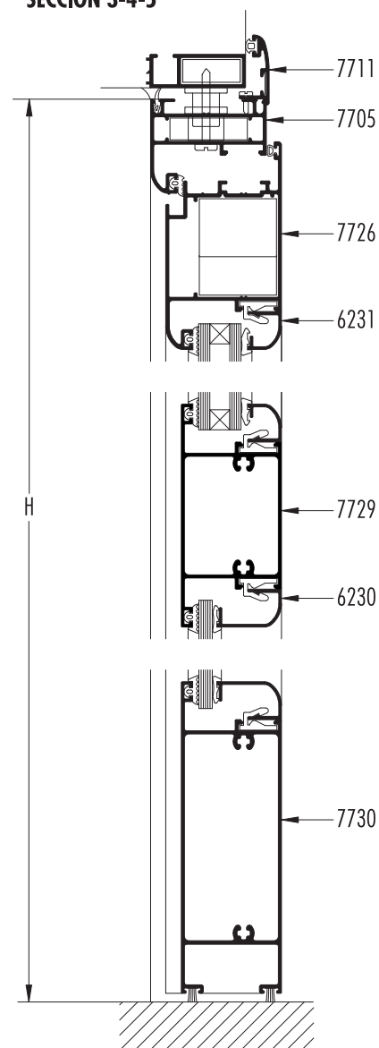
SECCION 3-4-5
