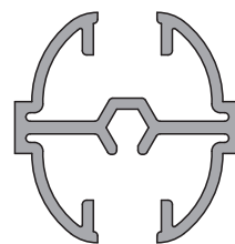
6268 0,429 kg/m
