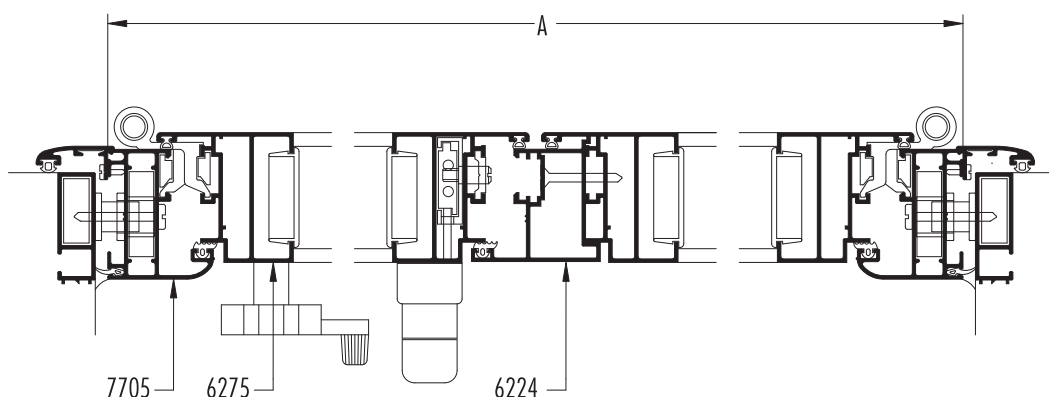
SECCION 1-2-3
