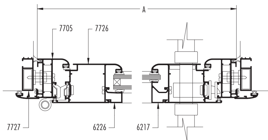
SECCION 1-2
