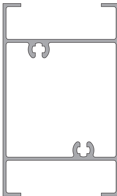
6276 1,301 kg/m
