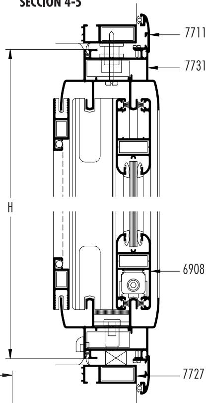
SECCION 4-5
