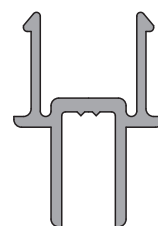
6246 0,292 kg/m
