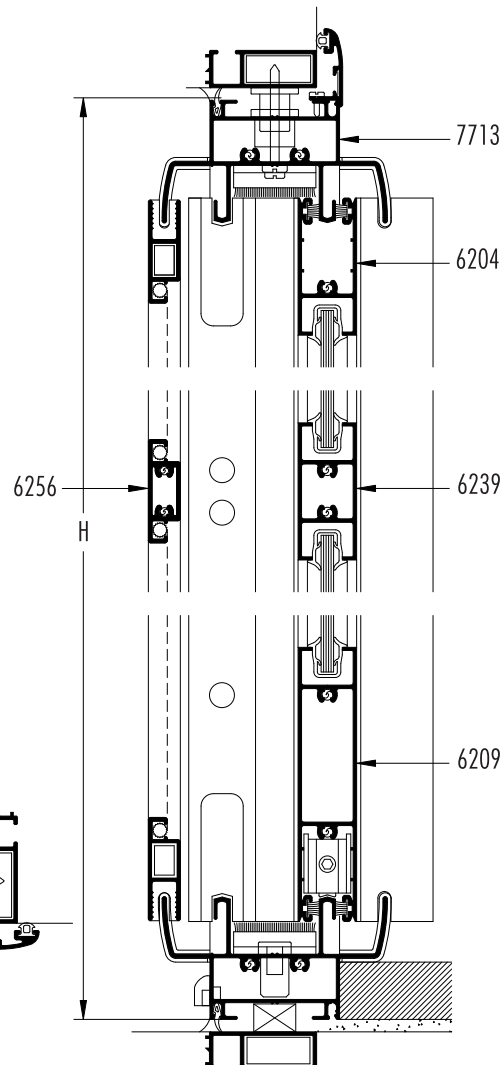
SECCION 4-7-8
